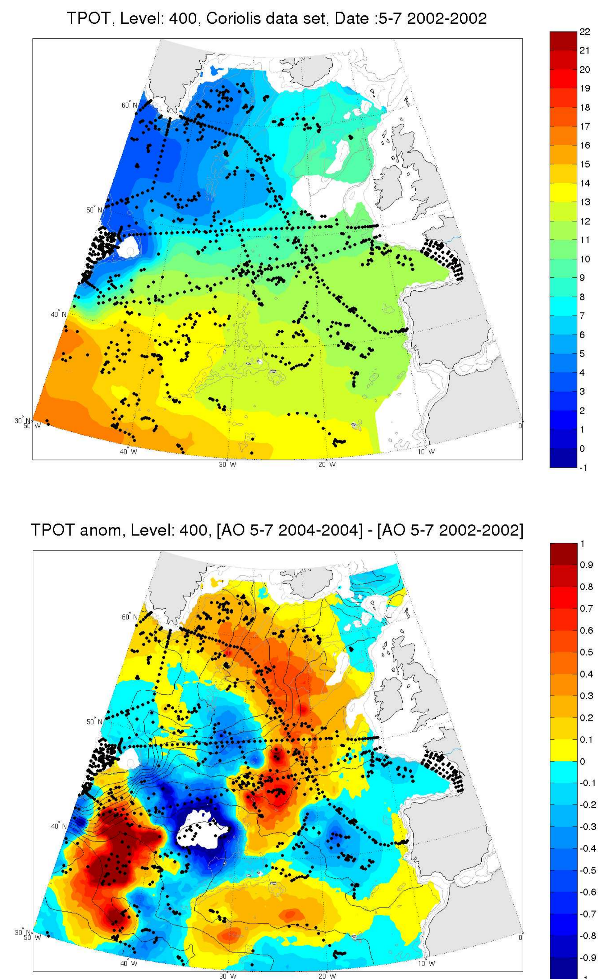
FIGURE 2: (a) Carte horizontale de température potentielle à 400 m reconstruite par analyse objective sur la période mai-juillet 2002. (b) Différence entre les températures potentielles à 400 m reconstruites par analyse objective sur la période mai-juillet 2004 et la période mai-juillet 2002 (V. Thierry).
