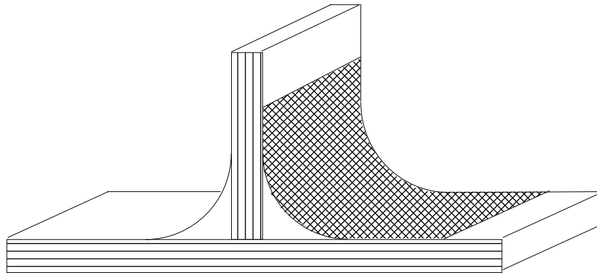
Schéma 6 : Joint-congé basse densité renforcé par un stratifié Bi-axial (-45° / +45°)
