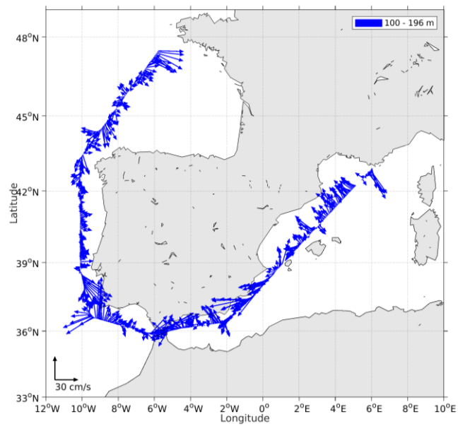
Figure 6- Vecteurs du courant de la section 1 de 100 à 200 m
