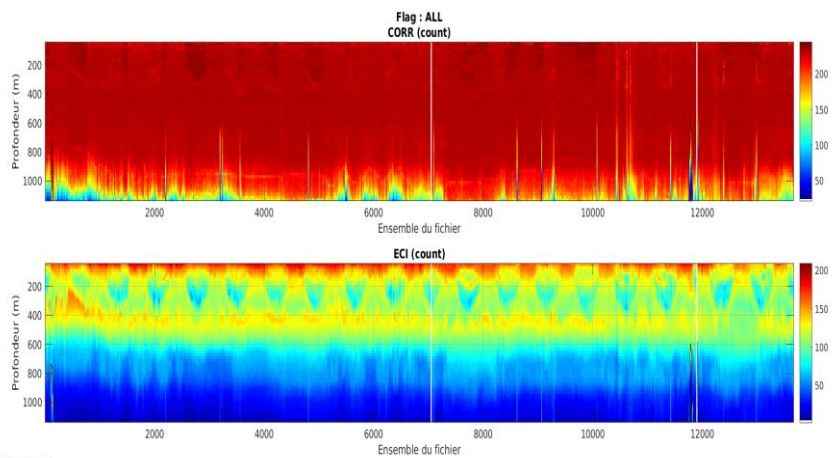
Figure 14 – Indicateur de corrélation (graphe haut) et intensité de l'écho rétro-diffusé (graphe bas) pour tous les flags qualité
