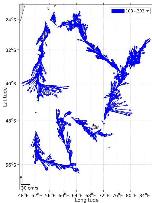
Figure 7- Vecteurs du courant de 100 à 300 m
